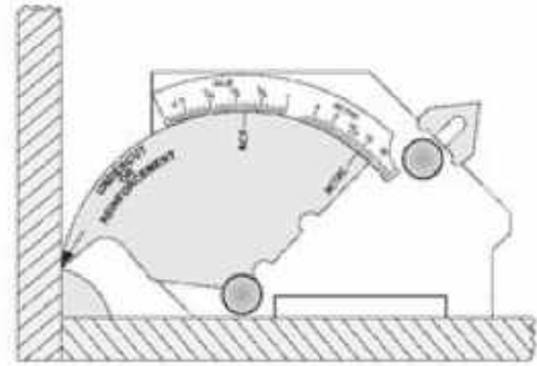
Fillet leg length
